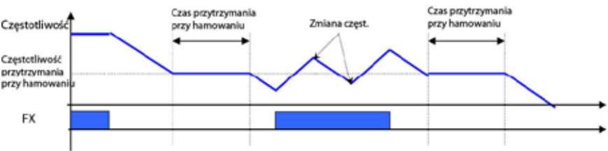
Wykres pracy przy hamowaniu
