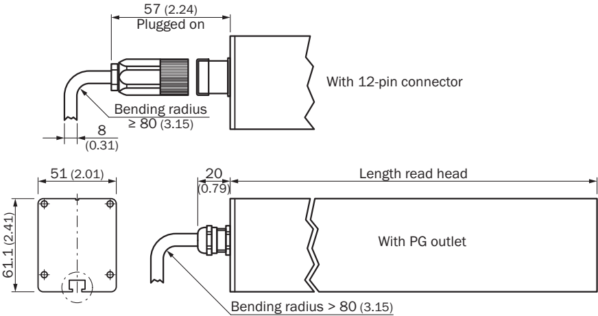
RYSUNEK WYMIAROWY GŁOWICA ODCZYTUJĄCA SSI
