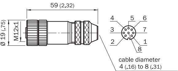
Rysunek wymiarowy
