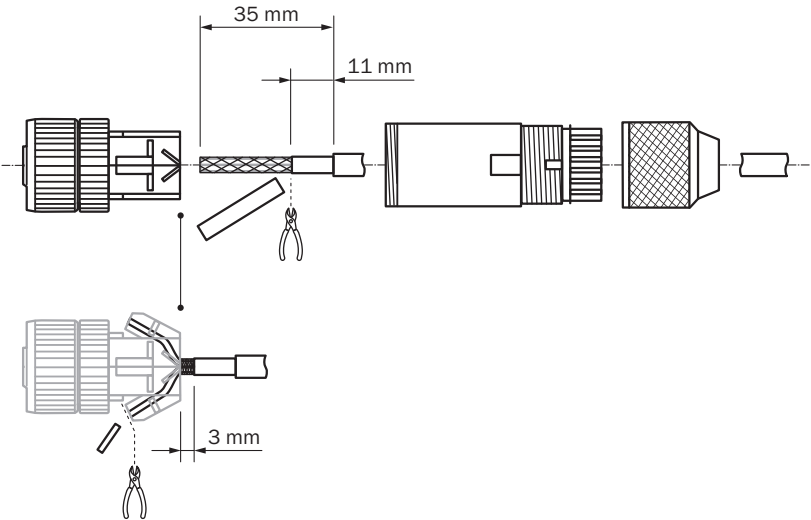
Rysunek montażowy
