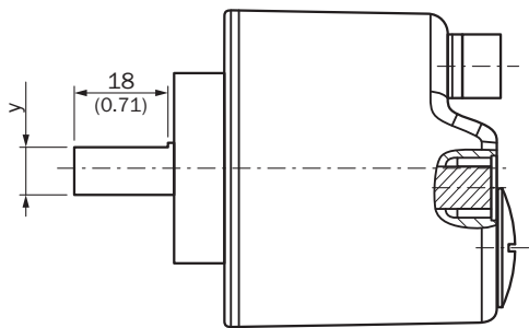
Rysunek wymiarowy Wałek pełny, z kołnierzem zaciskowym
