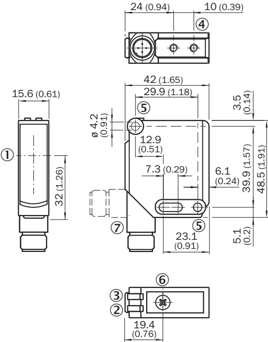
RYSUNEK WYMIAROWY WL12-3, WSE12-3
