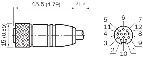
Rysunek wymiarowy (Wymiary w mm)
