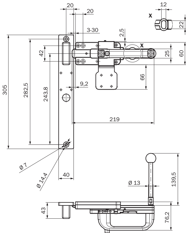
Rysunek wymiarowy (Wymiary w mm)
