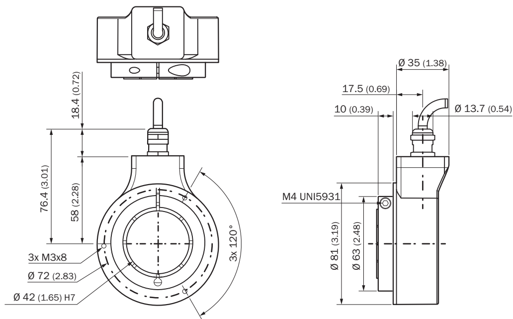
Rysunek wymiarowy Wielkość otworu 42 mm, przewód
