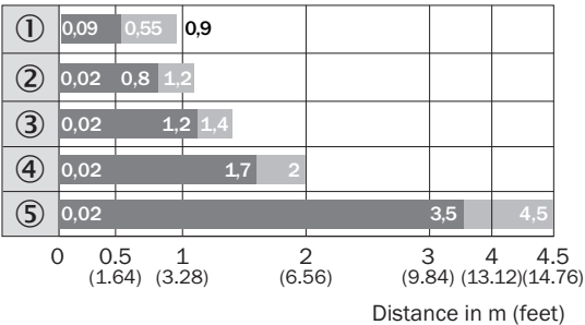
WYKRES ZASIĘGU WYKRYWANIA WLG4-3 Z FILTREM POLARYZACYJNYM
