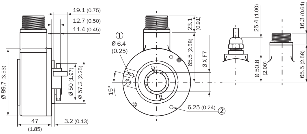
Rysunek wymiarowy
