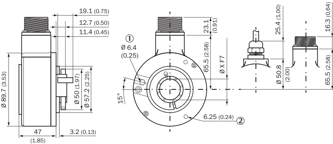
Wymiary w mm ① kołek pasowany ② głębokość
