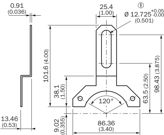
Wymiary w mm ① otwór podłużny T1 do śruby 3/8"
