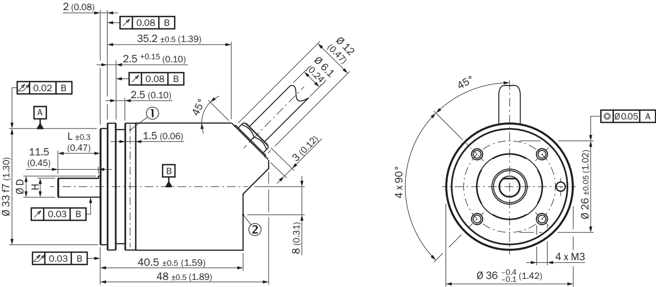
RYСУNEK WYMIAROWY WAŁEK, MOCOWANIE NA SERWOKOŁNIERZU, PRZEWÓD
