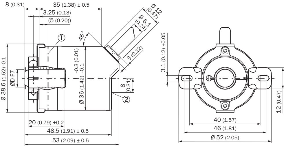
RYСУNEK WYMIAROWY WERSJA Z OTWOREM NIEPRZELOTOWYM, PRZEWÓD
