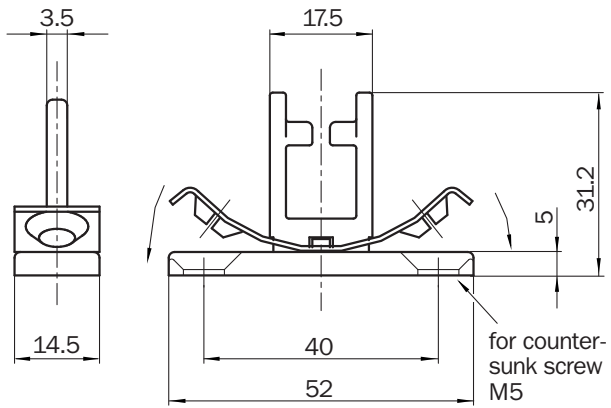
Rysunek wymiarowy (Wymiary w mm)
