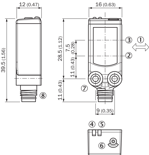
Rysunek wymiarowy (Wymiary w mm)
