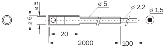
Rysunek wymiarowy (Wymiary w mm)
