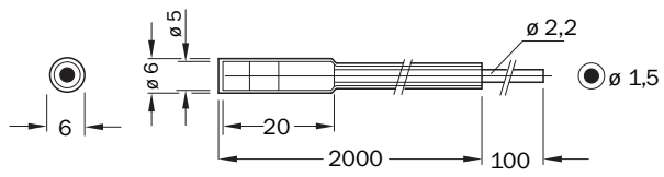
Rysunek wymiarowy (Wymiary w mm)
