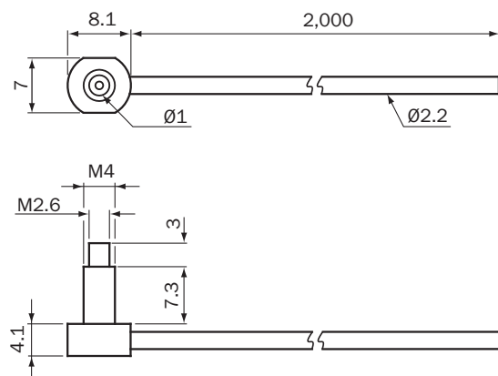
Rysunek wymiarowy (Wymiary w mm)
