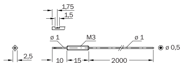
Rysunek wymiarowy (Wymiary w mm)
