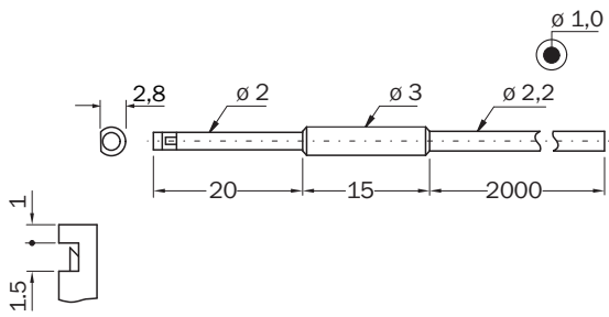
Rysunek wymiarowy (Wymiary w mm)
