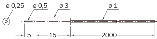
Rysunek wymiarowy (Wymiary w mm)
