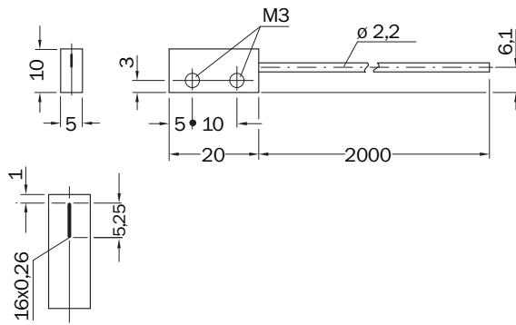
Rysunek wymiarowy (Wymiary w mm)
