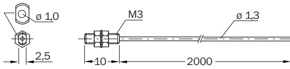
Rysunek wymiarowy (Wymiary w mm)
