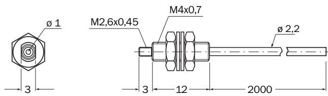
Rysunek wymiarowy (Wymiary w mm)
