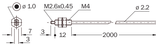
Rysunek wymiarowy (Wymiary w mm)
