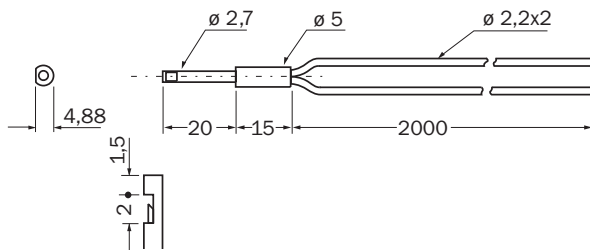
Rysunek wymiarowy (Wymiary w mm)
