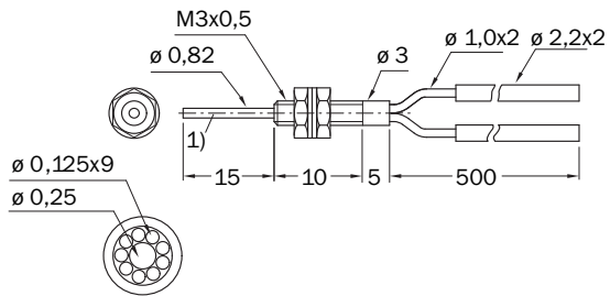
Rysunek wymiarowy (Wymiary w mm)
