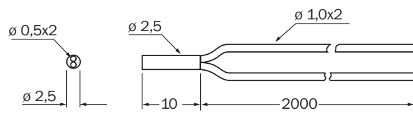
Rysunek wymiarowy (Wymiary w mm)
