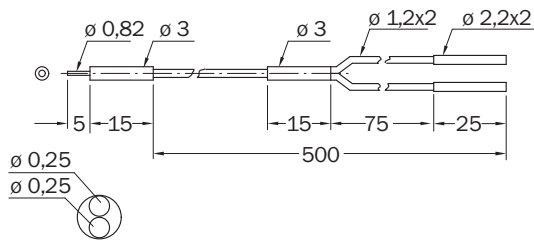
Rysunek wymiarowy (Wymiary w mm)
