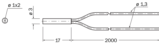
Rysunek wymiarowy (Wymiary w mm)
