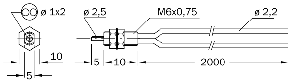
Rysunek wymiarowy (Wymiary w mm)
