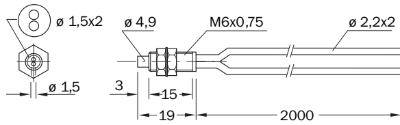
Rysunek wymiarowy (Wymiary w mm)
