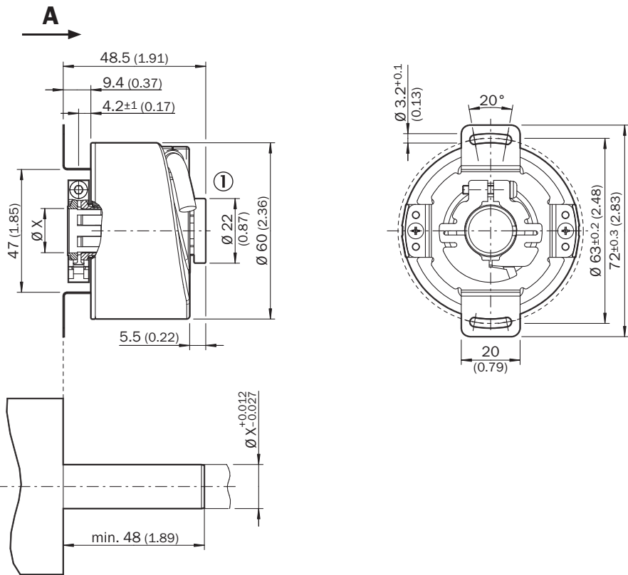
RYСУNEK WYMIAROWY OTWÓR PRZELOTOWY, ZACISK Z TWORZYWA SZTUCZNEGO, PRZEWÓD
