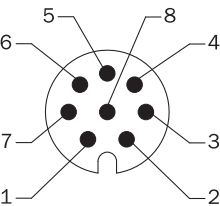
widok wtyczki urządzenia M12 na enkoderze
