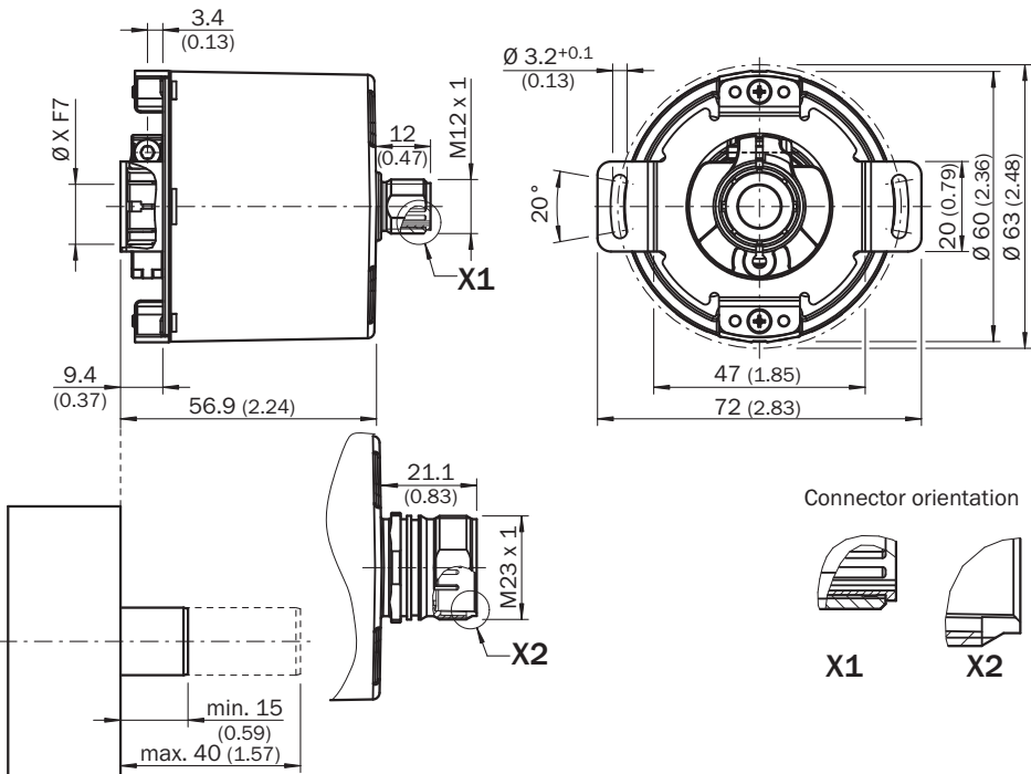
Wymiary w mm Tolerancje ogólne wg DIN ISO 2768-mk
