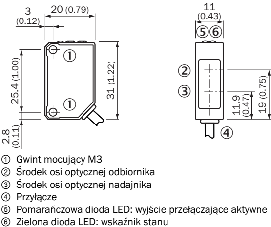
Rysunek wymiarowy (Wymiary w mm)
