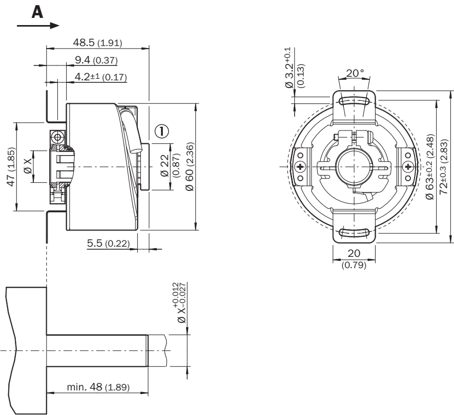
Wymiary w mm Tolerancje ogólne wg DIN ISO 2768-mk
